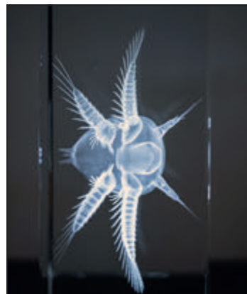
3D-Modell der Naupiluslarve eines ca 410 Millionen Jahre alten Krebses
